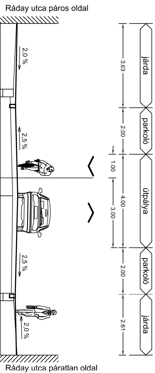
Ráday utca D-D metszet
