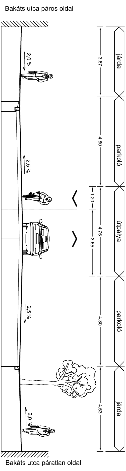
Bakáts utca I. A-A metszet
