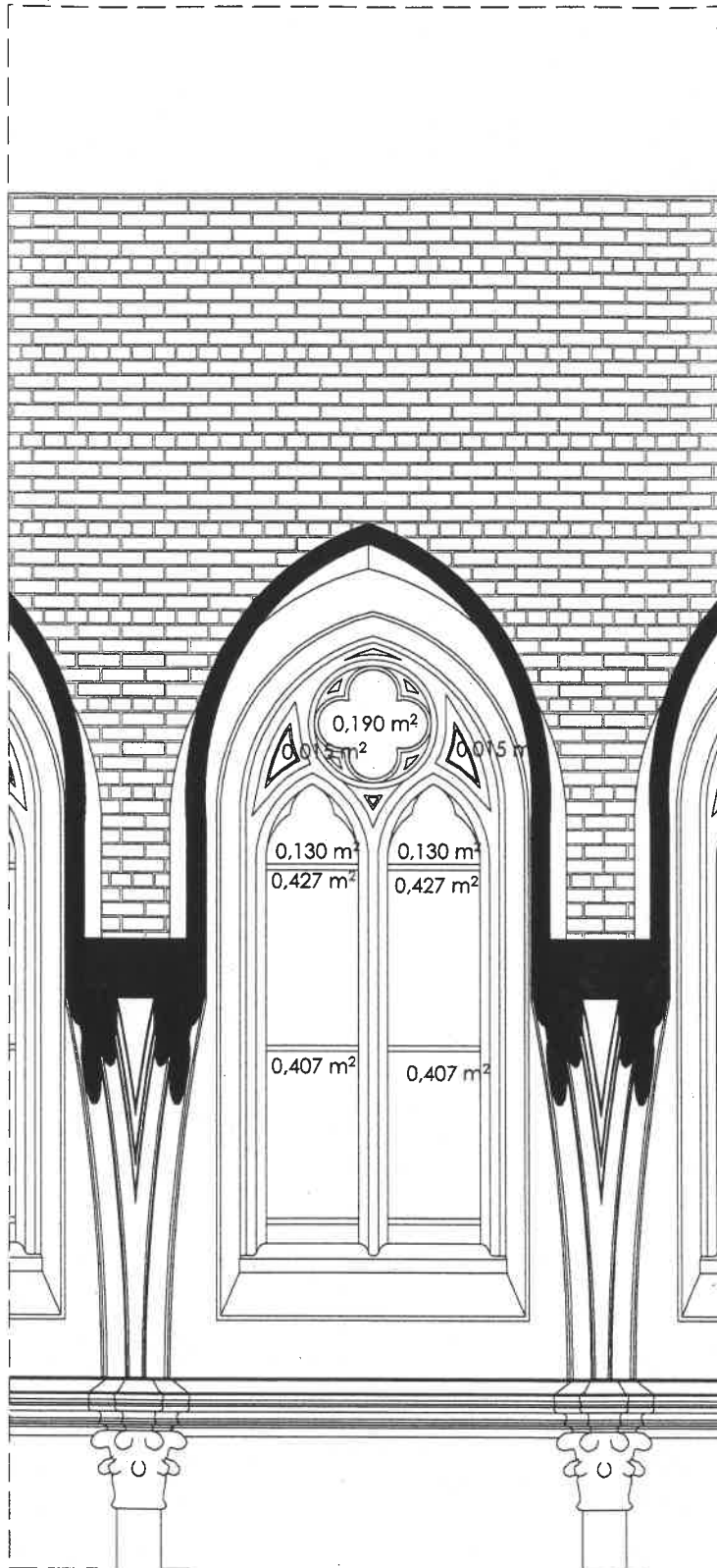
A-208 Ablak (025 Szentély felől)
